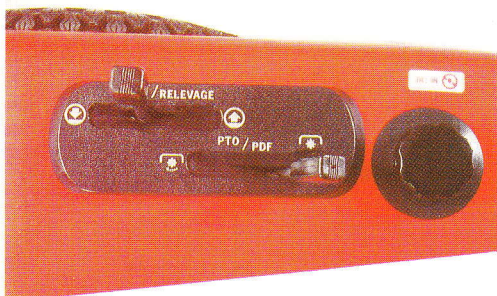
Hydraulische koppeling aftakas en hefinrichting.
